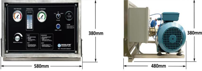
90-160-200 LİTRE/SAAT MODEL ÖLÇÜLERİ
