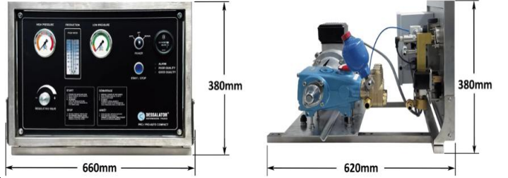
300 LİTRE/SAAT MODEL ÖLÇÜLERİ
